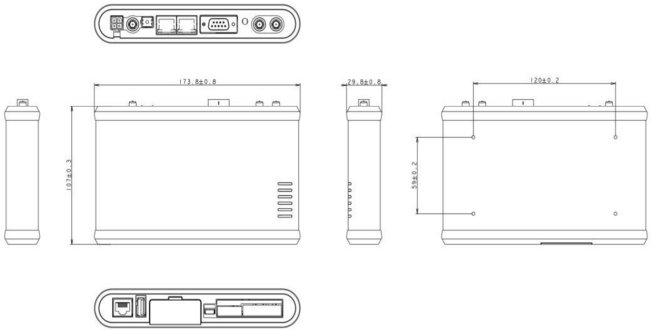
図 5 KILS22 外形
