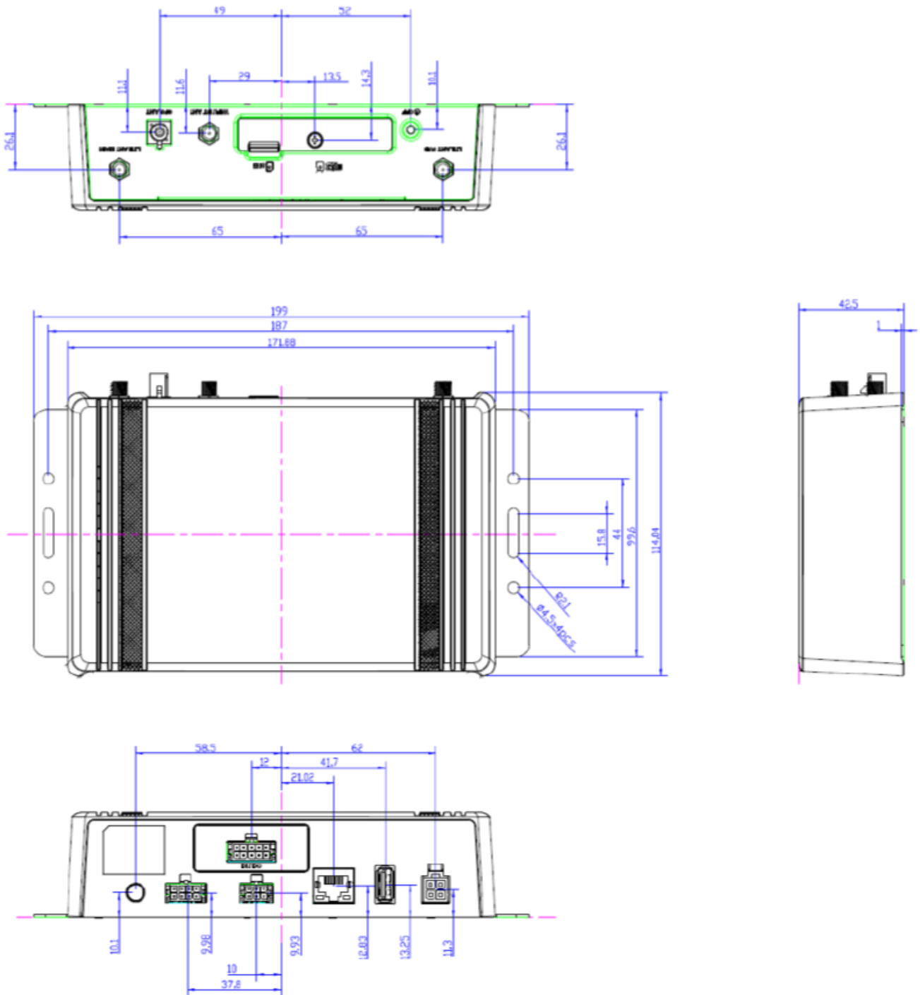
図 4 KILC12-*外形
