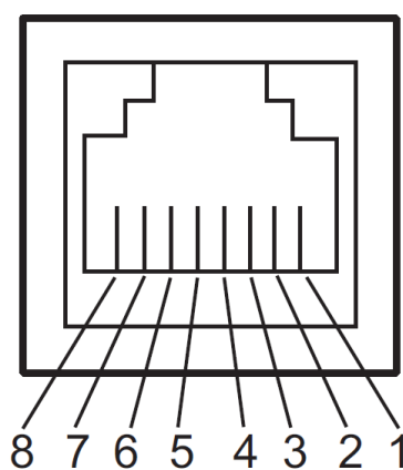
図 8 コネクタ
