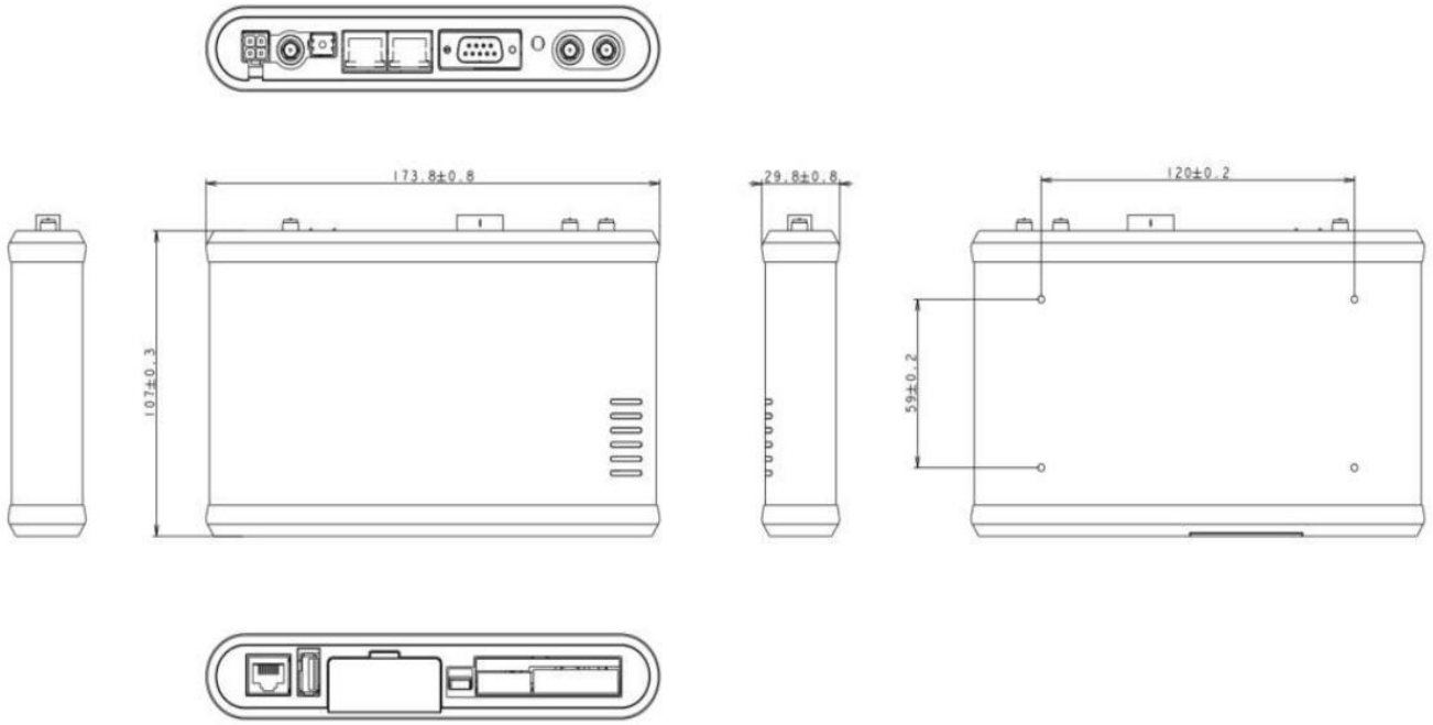
图 5 KILS22 外形
