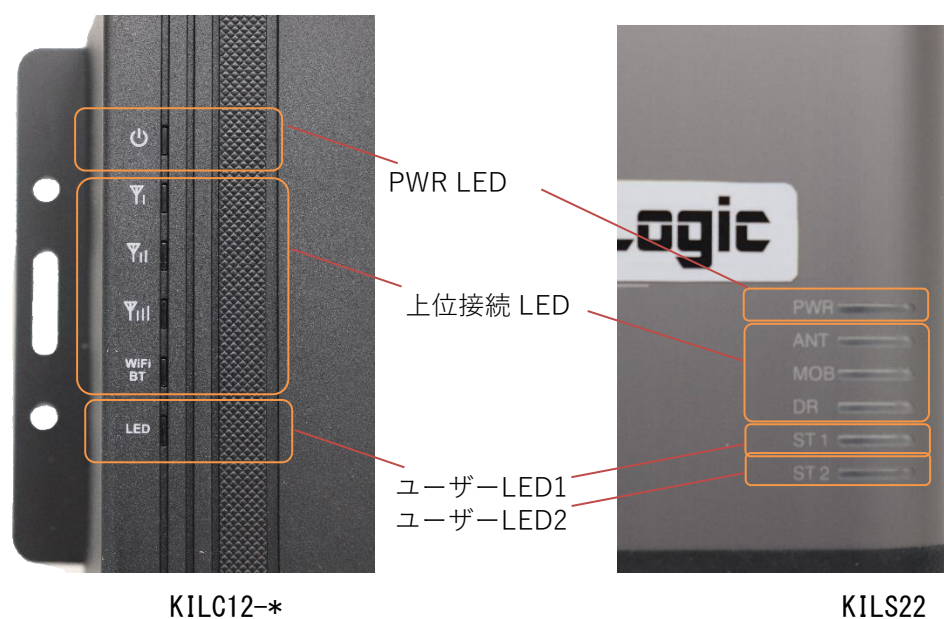
図 10 LED 配置
