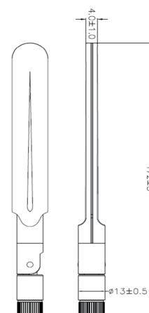
【LTE/3Gアンテナ】
